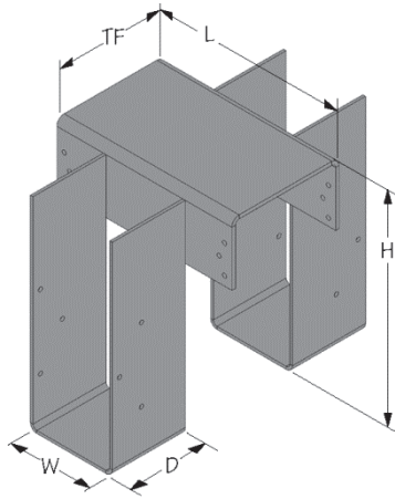
KGLS (KHGLS similar)
