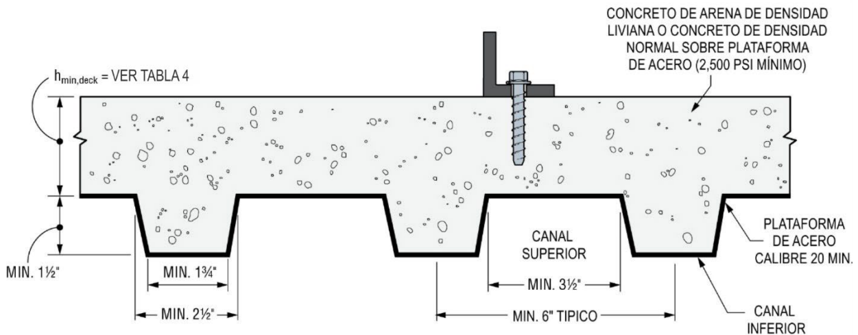
FIGURA 5—INSTALACIÓN DE ANCLAJES DE TORNILLOS DE ¼ DE PULGADA, 3/8 DE PULGADA y 1/2 DE PULGADA DE DIÁMETRO DEL VÁSTAGO EN LA PARTE SUPERIOR DE ENSAMBLAJES DE PISOS Y TECHOS DE PLATAFORMAS DE ACERO PERFILADAS RELLENAS DE CONCRETO (1 pulg = 25.4 mm)
