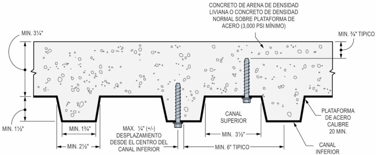
FIGURA 4—INSTALACIÓN DE ANCLAJES DE TORNILLOS DE ¼ DE PULGADA DE DIÁMETRO DEL VÁSTAGO Y SOPORTES DE VARILLAS ROSCADAS EN EL SOFITO SOBRE PLATAFORMAS DE ACERO PERFILADAS EN ENSAMBLAJES DE PISOS Y TECHOS (1 pulg = 25.4 mm)
